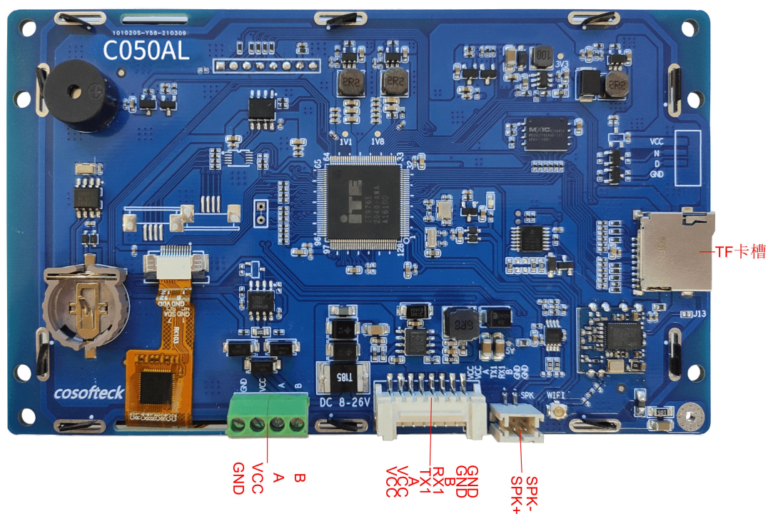
背面视图
