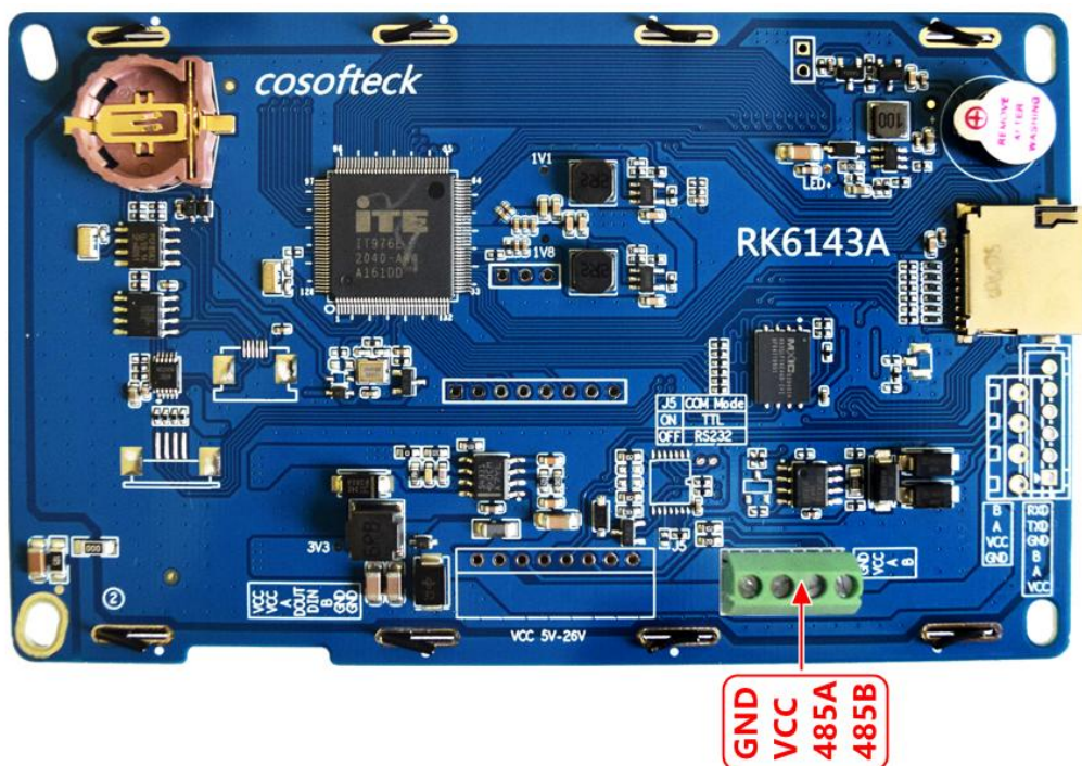
背面视图 (2)
