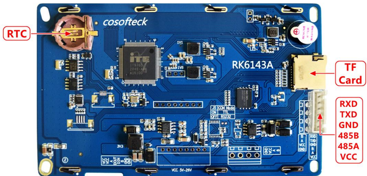
背面视图 (1)
