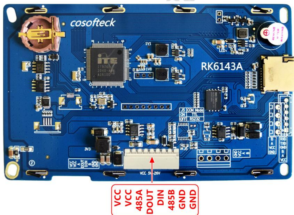
背面视图 (3)
