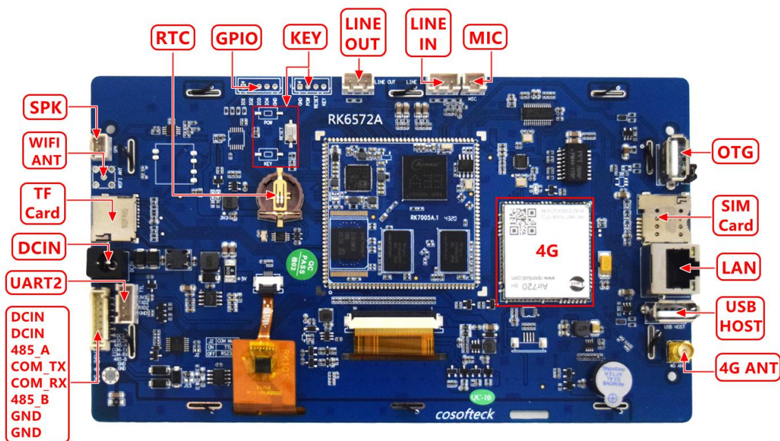
带 4G 功能背面视图
