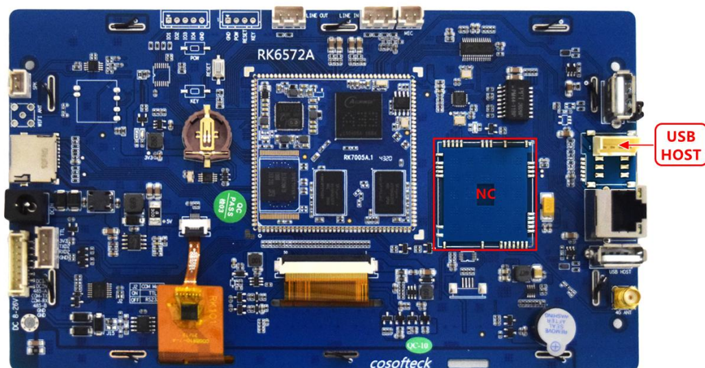
无 4G 功能背面视图
